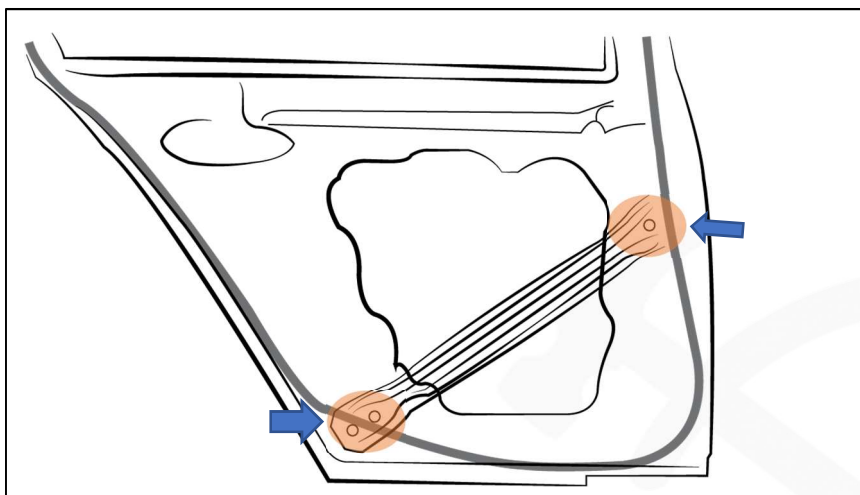
Bild: 1 – Beispiel Tür 5er BMW G31
