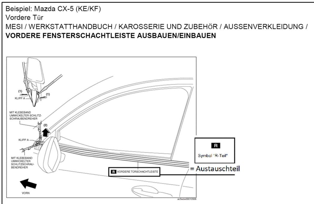
Bild 2: Auszug aus Reparaturleitfaden Mazda CX-5 mit Hinweis auf R-Teil „Fensterschachtleiste“
